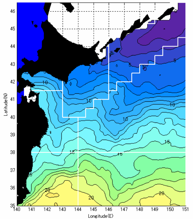
12月下旬予測水温分布図
