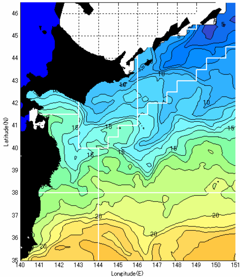
11月中旬予測水温分布図
