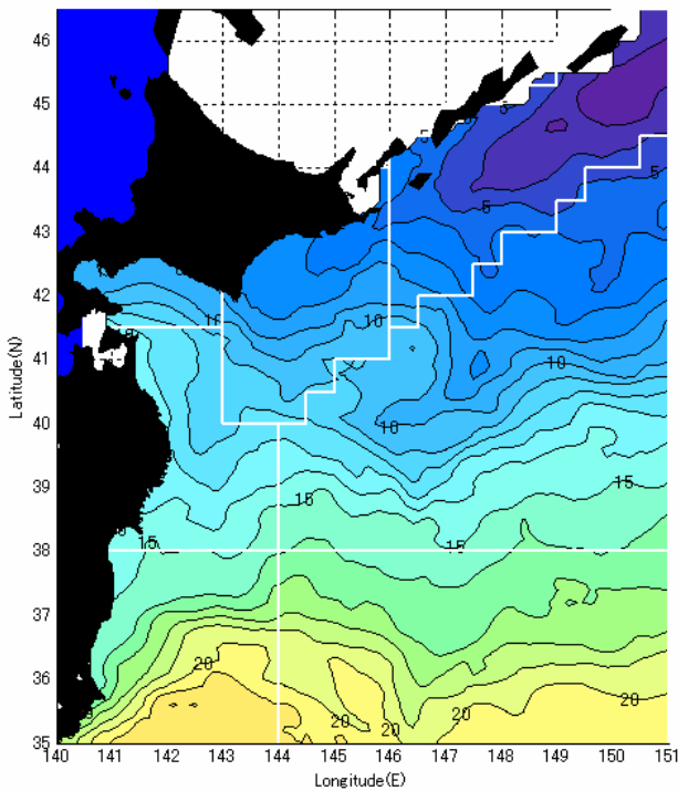
12月中旬予測水温分布図
