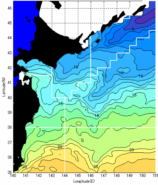
11月下旬予測水温分布図
