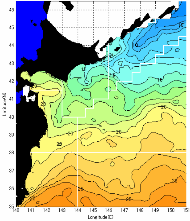
10月上旬予測水温分布図
