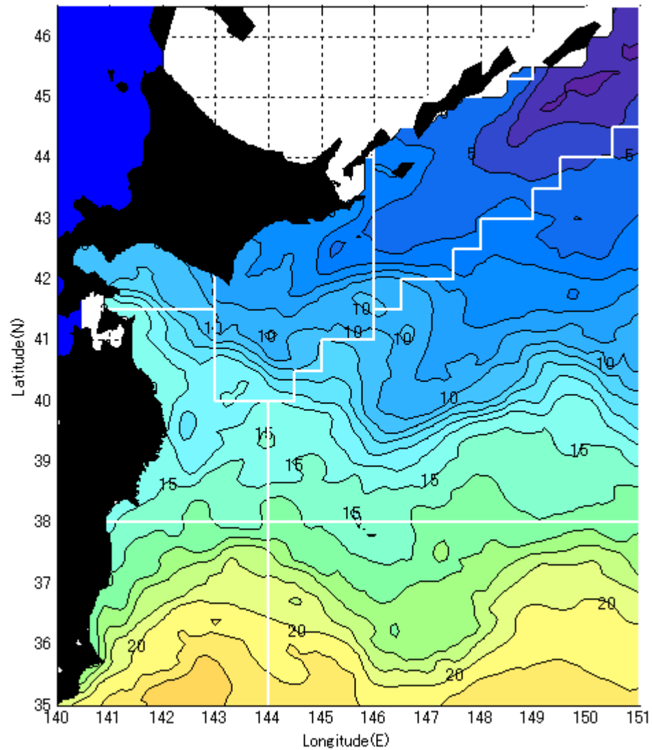
12月上旬予測水温分布図
