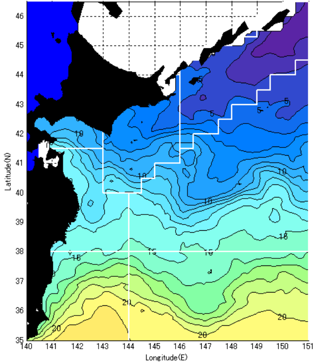
1月上旬予測水温分布図
