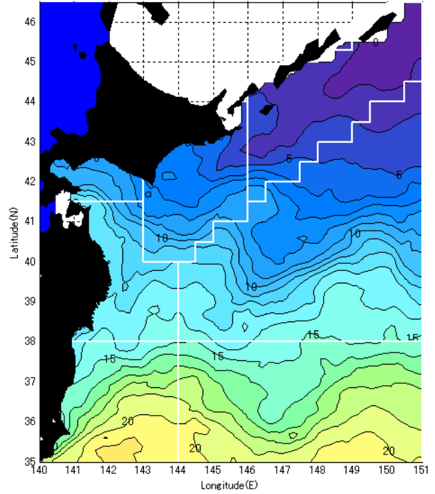
1月中旬予測水温分布図
